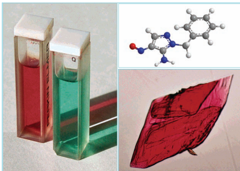
Disoluciones en metanol (rojo) y en acetato de etilo (verde) de un derivado de pirazol
