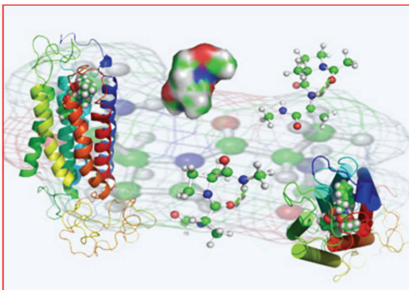
Diseño racional de fármacos asistido por ordenador
