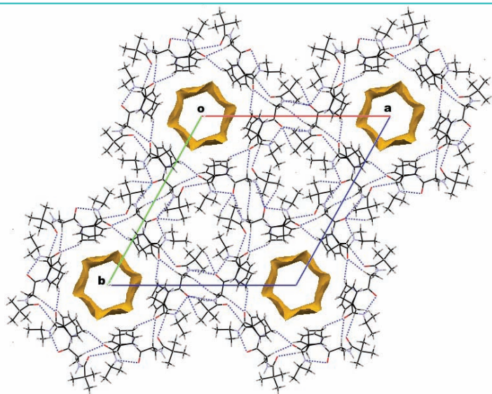
RAYOS X. Autoensamblaje de moléculas en forma de superficie porosa
